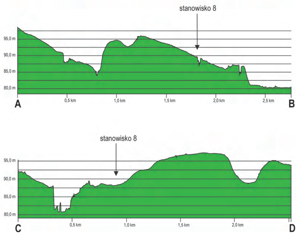
Ryc. 2. Numeryczny model terenu okolicy stanowiska 8 w Kleszewie z zaznaczeniem jego lokalizacji. Oprac.: T. Rakowski
